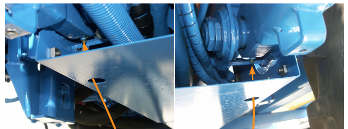
Support d'incorporeur ▲
