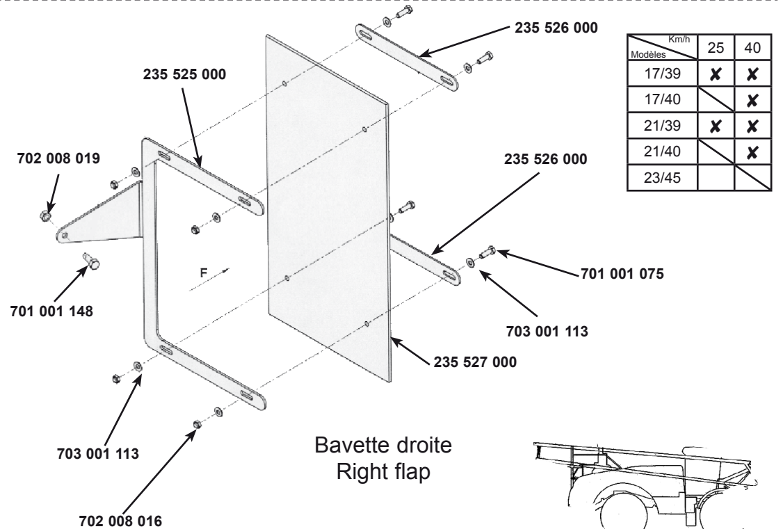
Bavette droite Right flap
