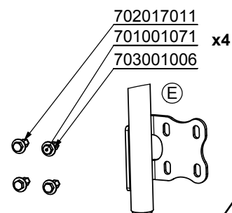
DÉTAIL E ECHELLE 1 : 4
