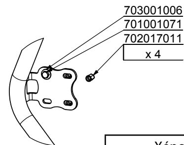
DÉTAIL D
