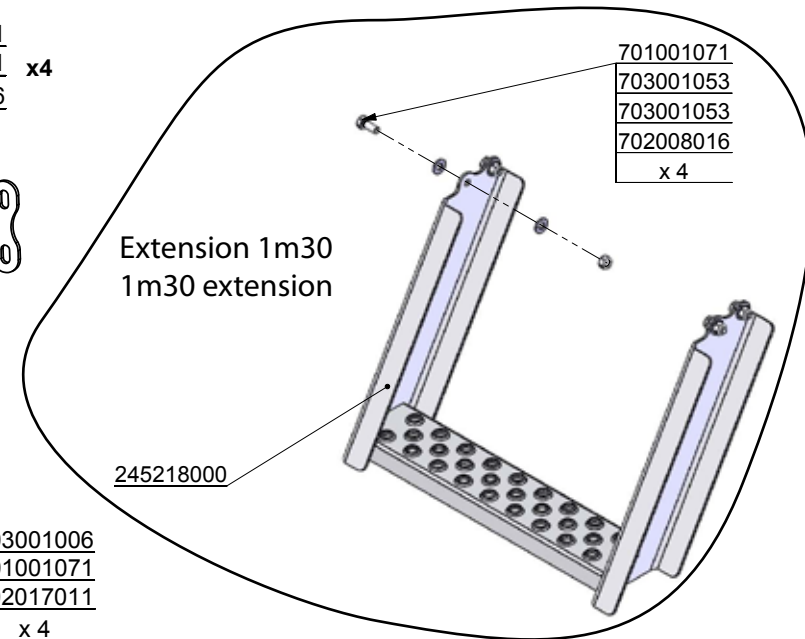
DÉTAIL E ECHELLE 1 : 4
