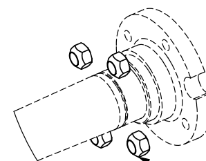
DÉTAIL B ECHELLE 1 : 3
